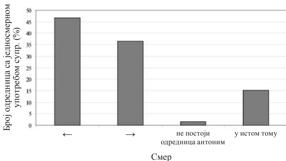
Слика 5: Процентуални приказ смера једносмерних квалификатора супр.
